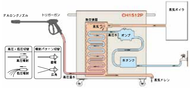
構造図
