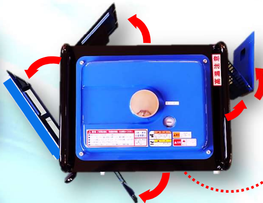
オイルドレン集中配置
