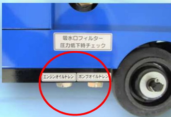
オイルドレン集中配置
