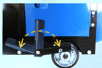
らくらく 車輪ストップ
