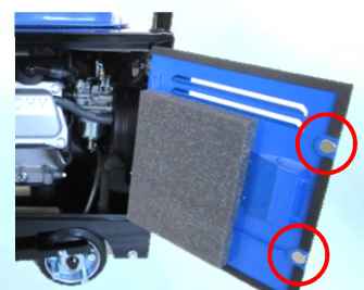
ネオジウム強力磁石採用
